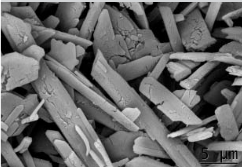
Imagen de cristales de yeso fino (gesso sottile) correspondientes a bases de preparación en obras de arte del S. XVI. Se aprecian con amplio detalle las fracturas en los cristales tabulares debido a eliminación de moléculas de agua, así como su transformación de fase producto de la calcinación por efecto de la temperatura
